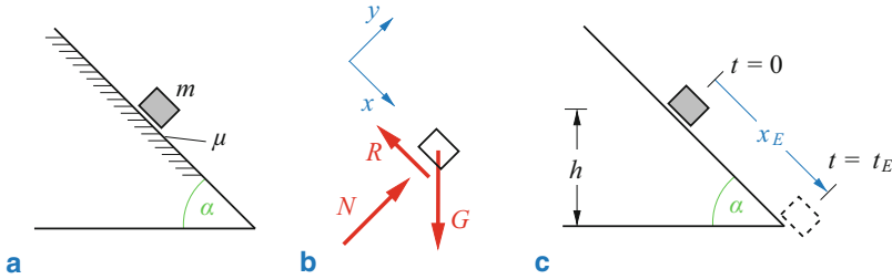
Abb. 1.15 Bewegung auf einer schiefen Ebene
