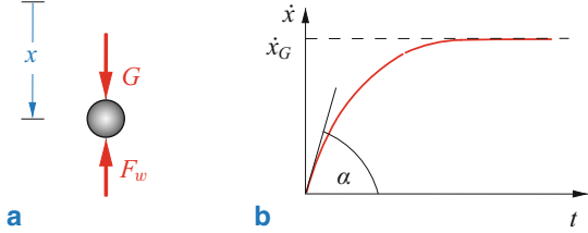
Abb. 1.16 Freier Fall mit Luftwiderstand
