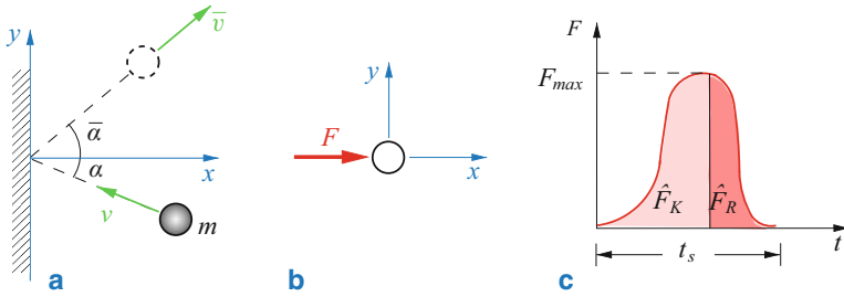
Abb. 1.17 Stoß gegen eine Wand
