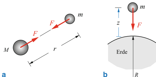
Abb. 1.25 Zum Gravitationsgesetz, Potential des Erdschwerefelds
