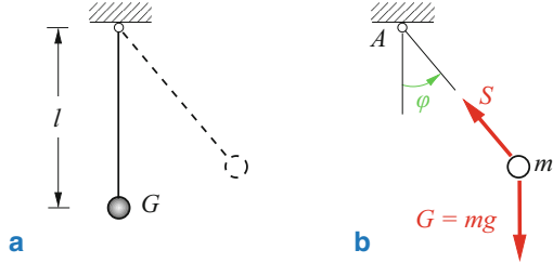
Abb. 1.22 Mathematisches Pendel
