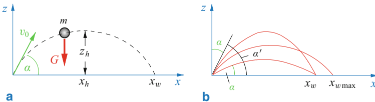
Abb. 1.13 Schiefer Wurf
