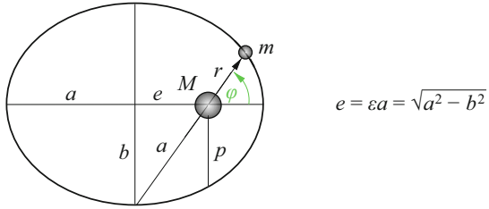
Abb. 1.26 Zum 1. Keplerschen Gesetz
