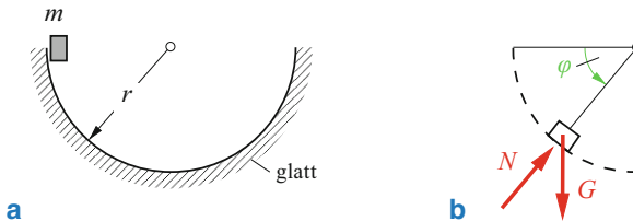
Abb. 1.14 Bewegung auf einer Kreisbahn
