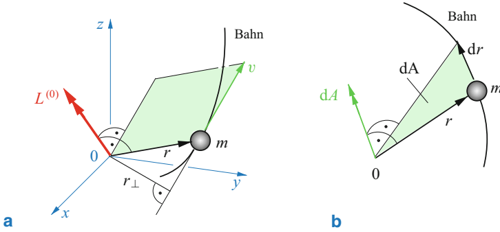
Abb. 1.19 Drehimpulsvektor
