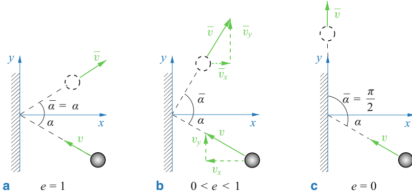
Abb. 1.18 Ideal-elastischer, teilelastischer, ideal-plastischer Stoß
